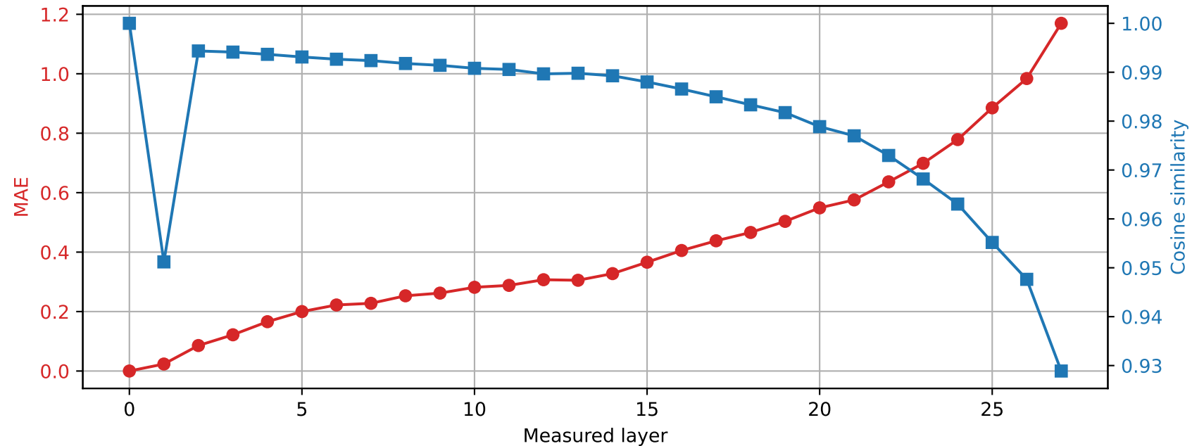
Llama-3.2-3B | Prompt 3 Spared layer 26 | Hybrid vs unquantized
