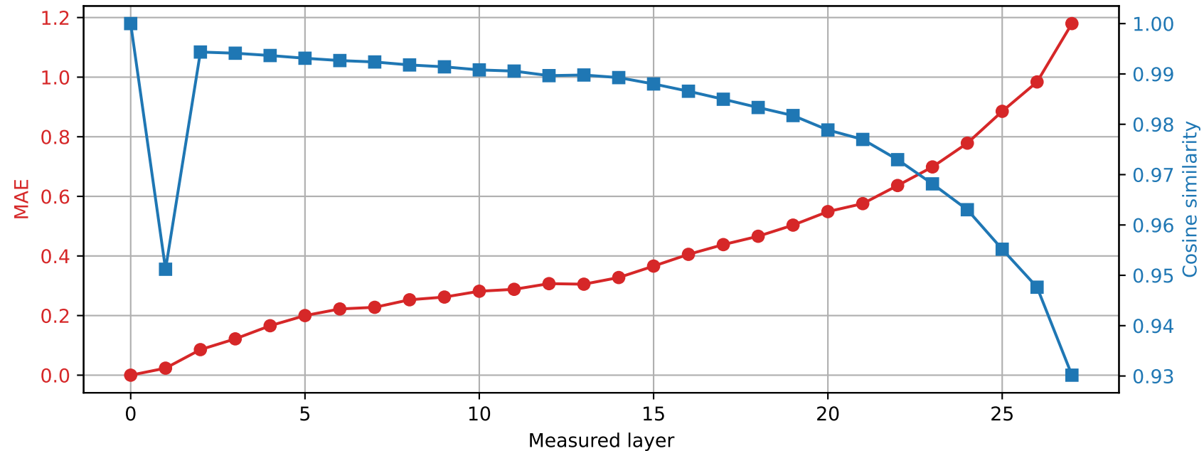
Llama-3.2-3B | Prompt 3 Spared layer 27 | Hybrid vs unquantized
