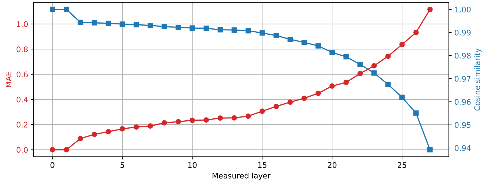
Llama-3.2-3B | Prompt 4 Spared layer 0 | Hybrid vs unquantized
