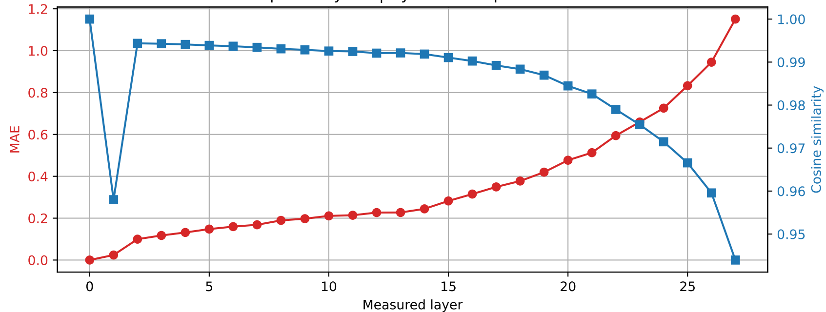
Llama-3.2-3B | Prompt 4 Spared layer 2 | Hybrid vs unquantized
