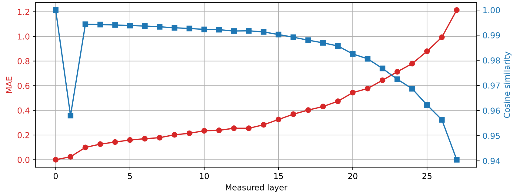
Llama-3.2-3B | Prompt 4 Spared layer 3 | Hybrid vs unquantized
