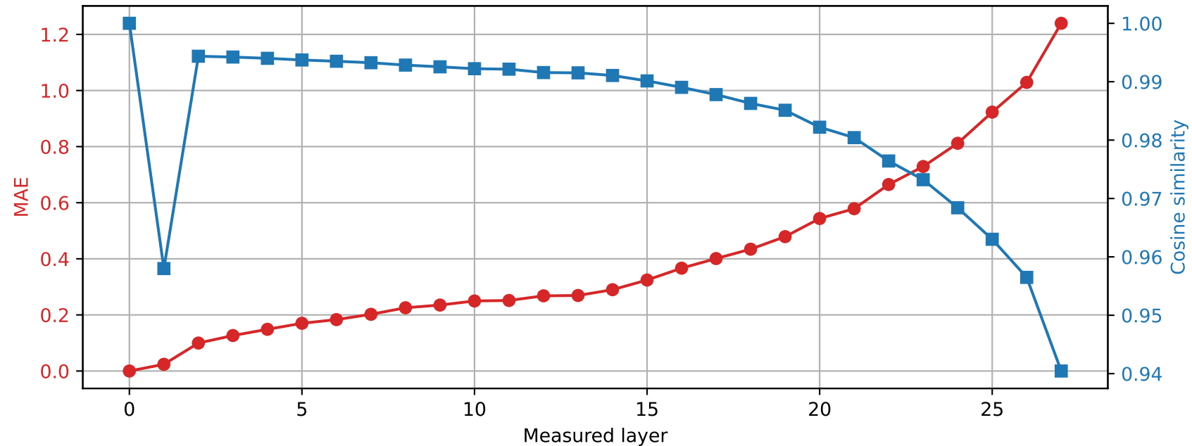
Llama-3.2-3B | Prompt 4 Spared layer 6 | Hybrid vs unquantized
