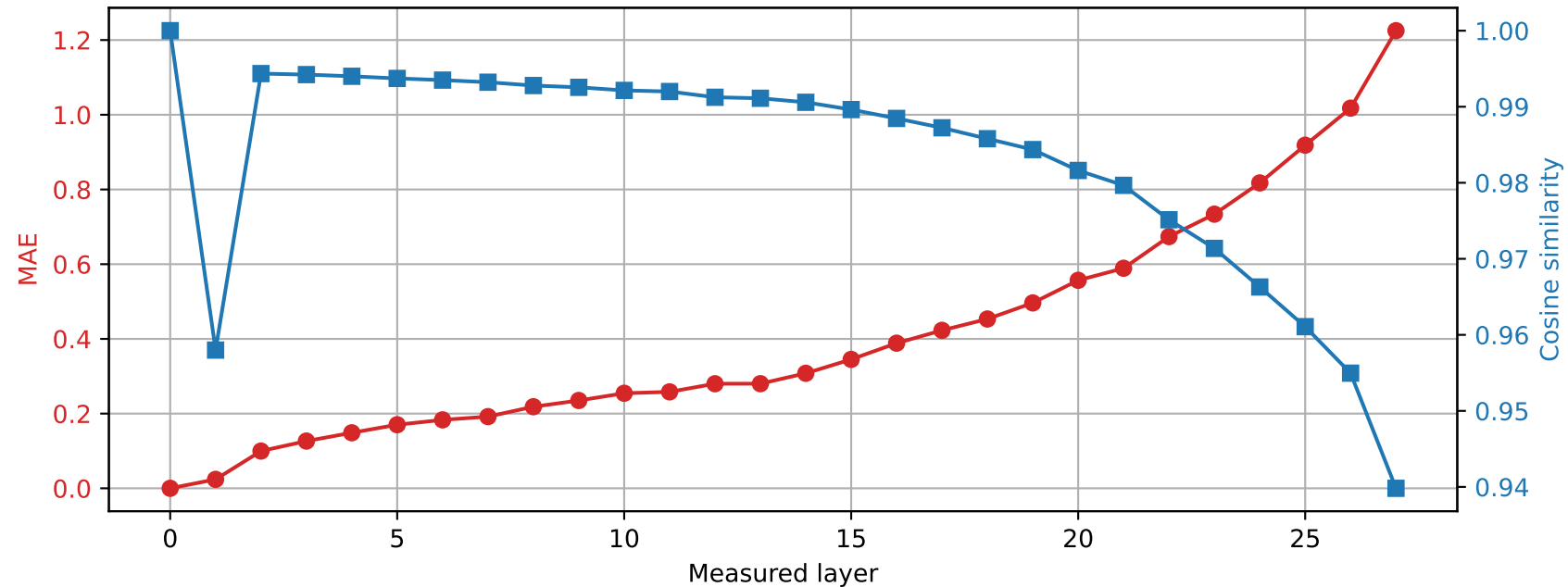
Llama-3.2-3B | Prompt 4 Spared layer 8 | Hybrid vs unquantized
