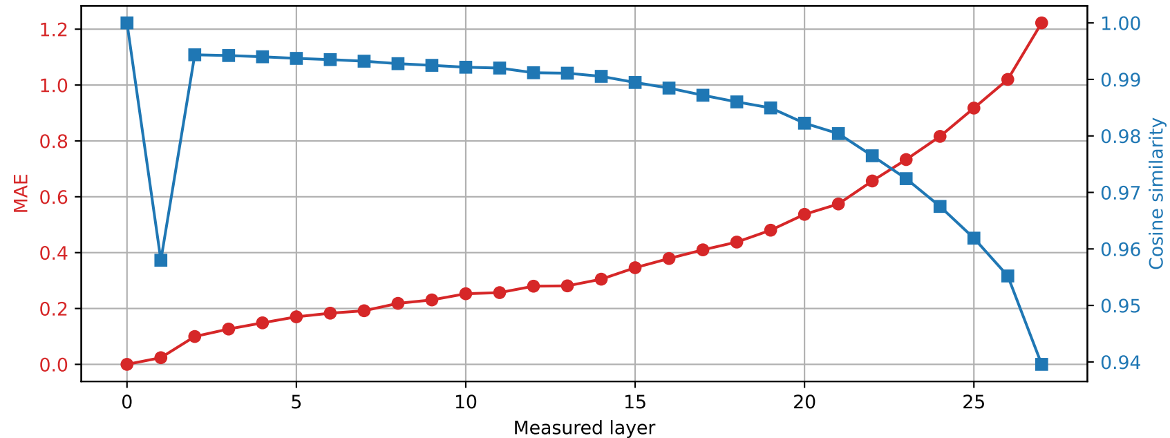
Llama-3.2-3B | Prompt 4 Spared layer 9 | Hybrid vs unquantized
