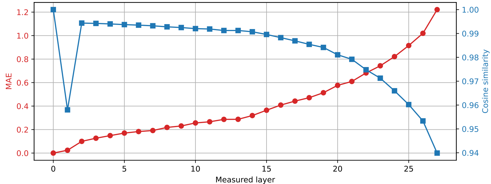
Llama-3.2-3B | Prompt 4 Spared layer 10 | Hybrid vs unquantized
