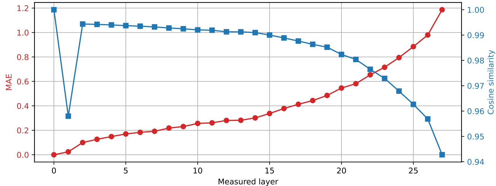
Llama-3.2-3B | Prompt 4 Spared layer 13 | Hybrid vs unquantized
