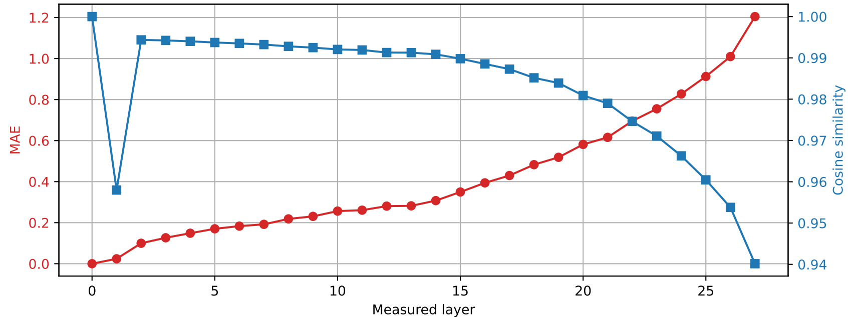
Llama-3.2-3B | Prompt 4 Spared layer 17 | Hybrid vs unquantized
