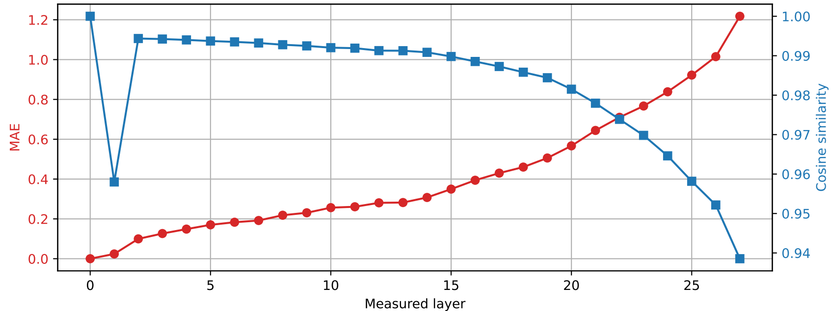
Llama-3.2-3B | Prompt 4 Spared layer 20 | Hybrid vs unquantized
