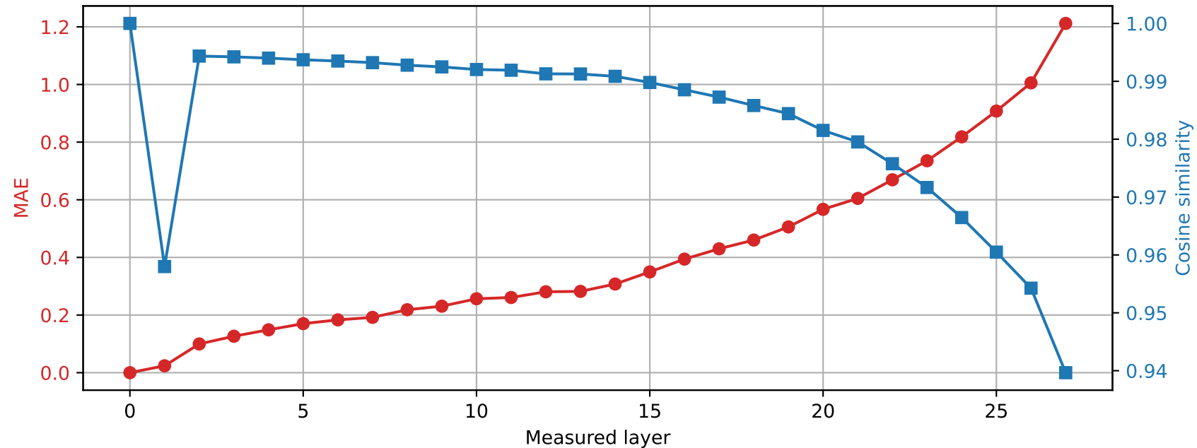
Llama-3.2-3B | Prompt 4 Spared layer 21 | Hybrid vs unquantized
