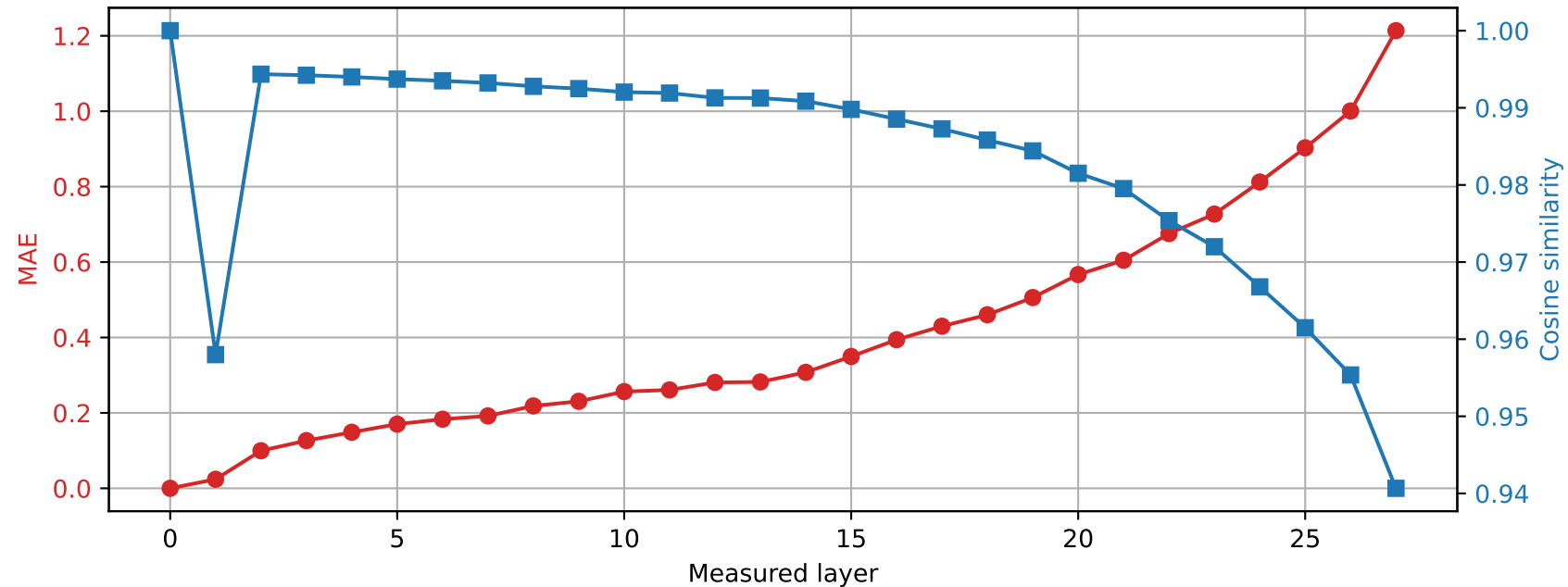
Llama-3.2-3B | Prompt 4 Spared layer 22 | Hybrid vs unquantized
