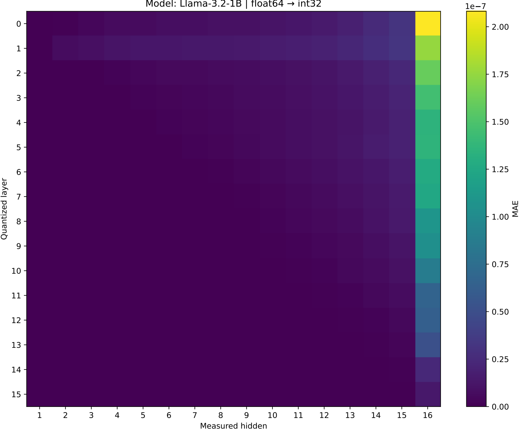
Model: Llama-3.2-1B | float64 → int32
