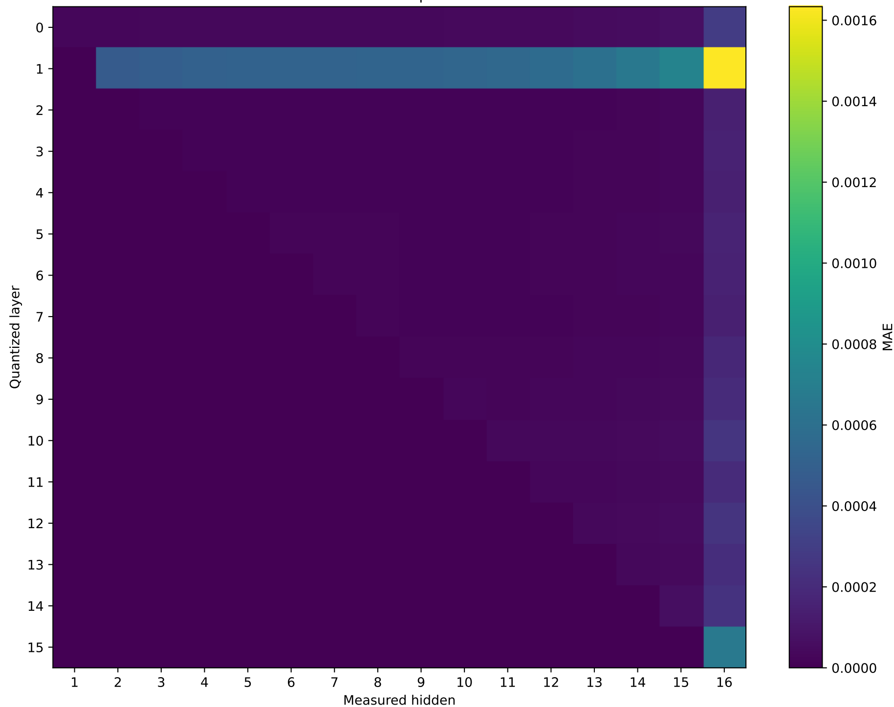
Model: Llama-3.2-1B | float32 → int16
