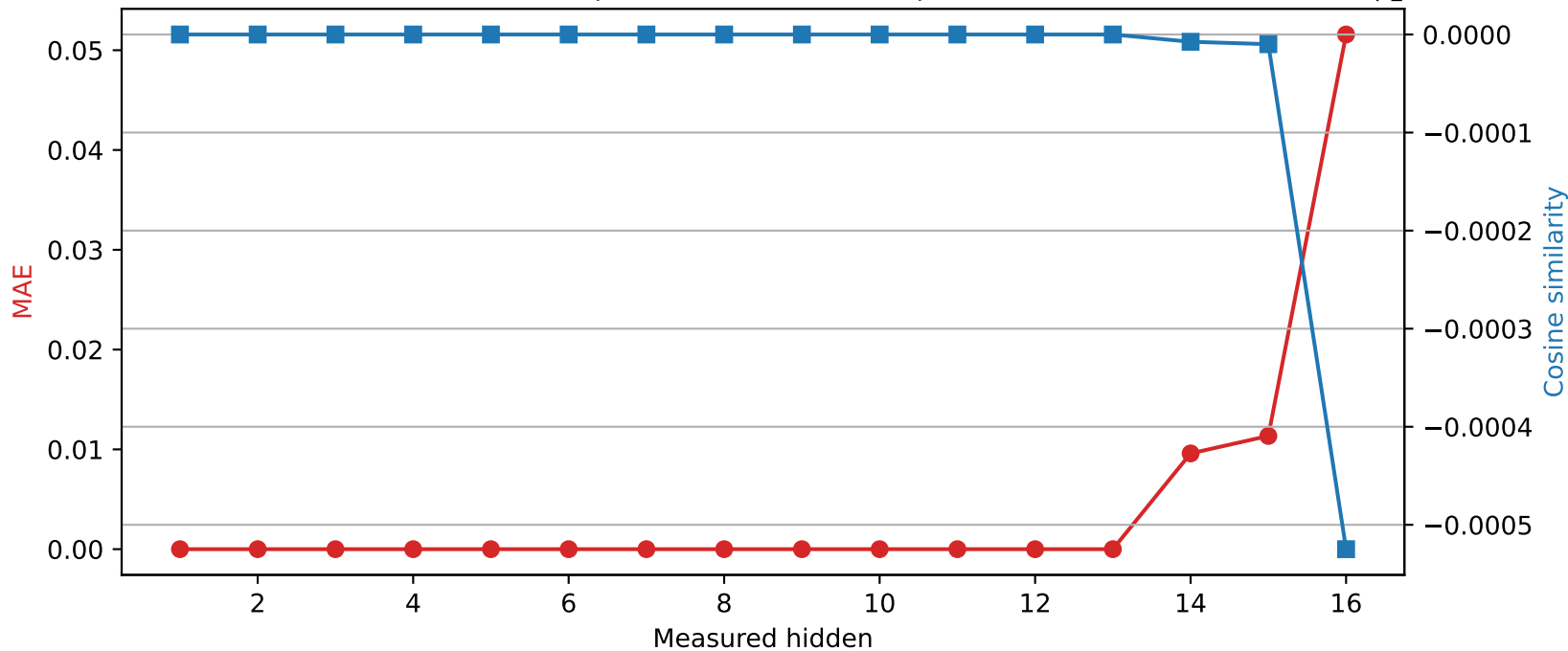
Llama-3.2-1B | Quantized layer 13 | float16 \rightarrow int8
