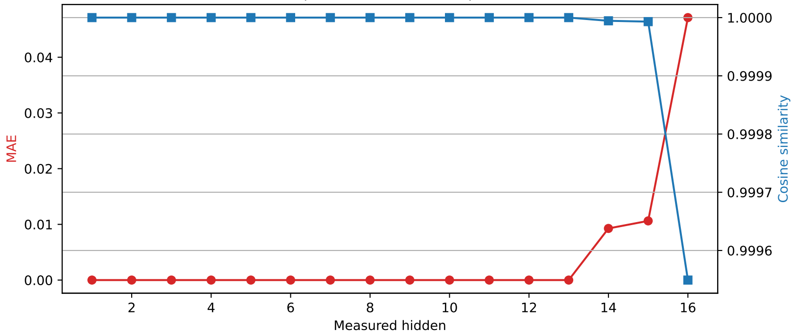
Llama-3.2-1B | Quantized layer 13 | float16 \rightarrow int8
