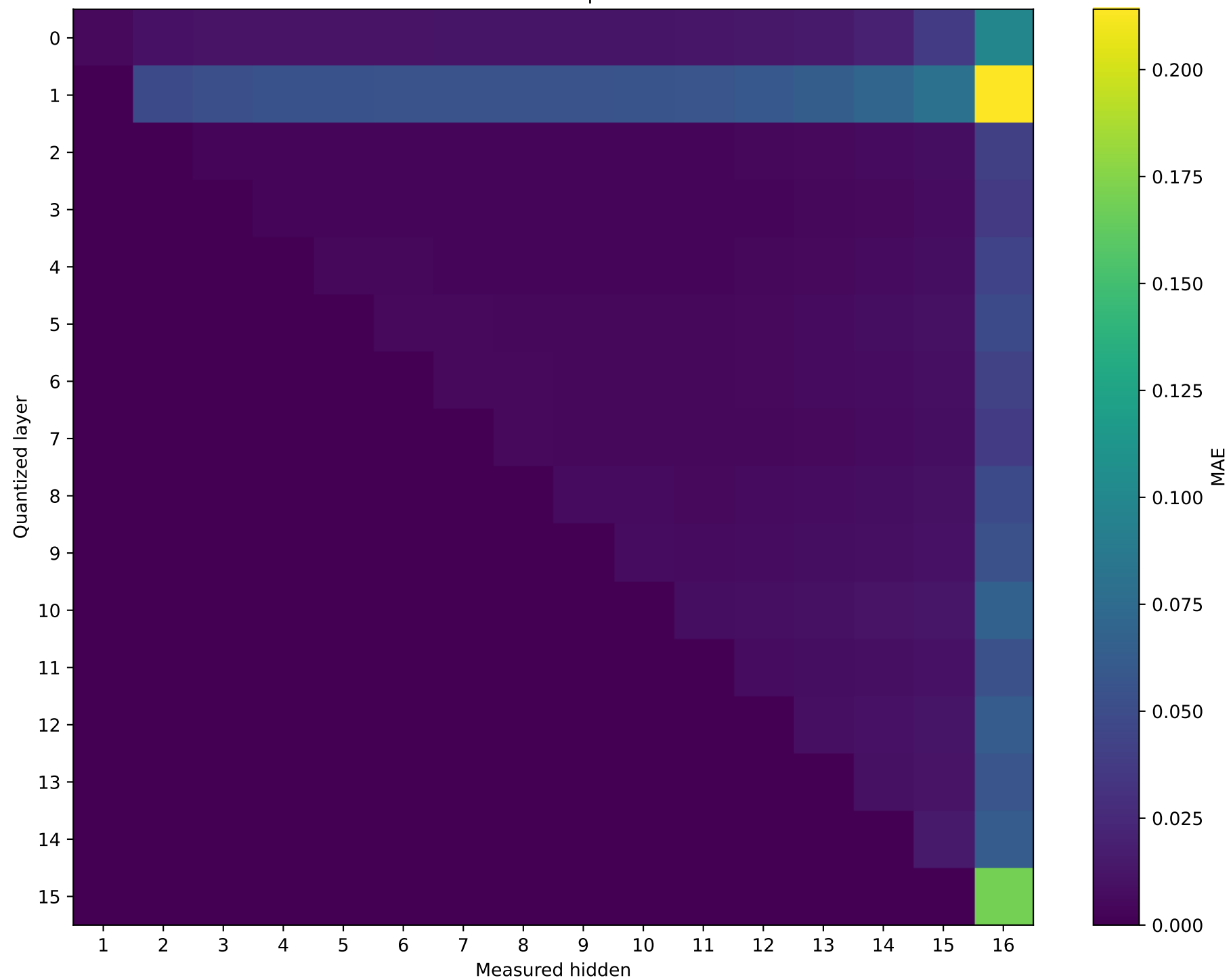
Model: Llama-3.2-1B | float32 \rightarrow int8
