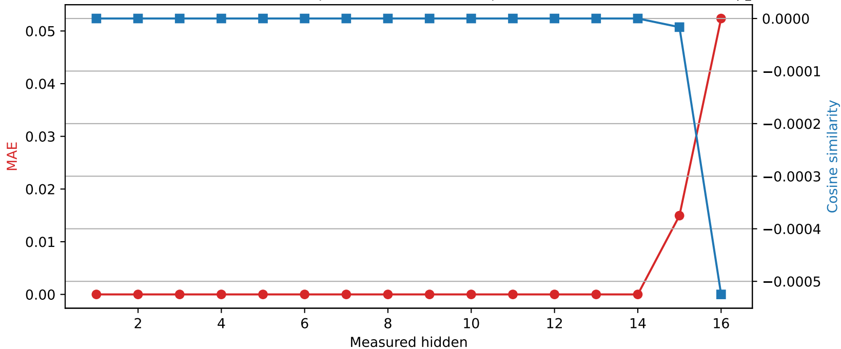
Llama-3.2-1B | Quantized layer 14 | float32 \rightarrow int8
