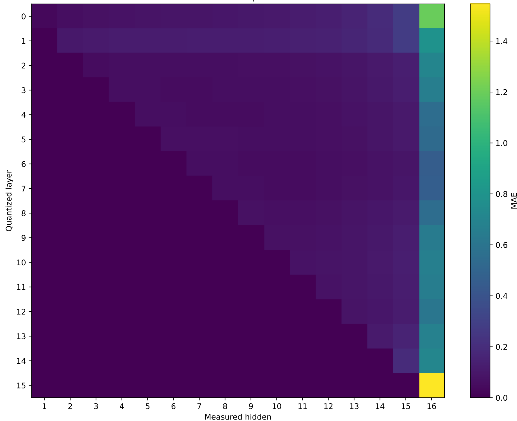
Model: Llama-3.2-1B | float16 \rightarrow int4
