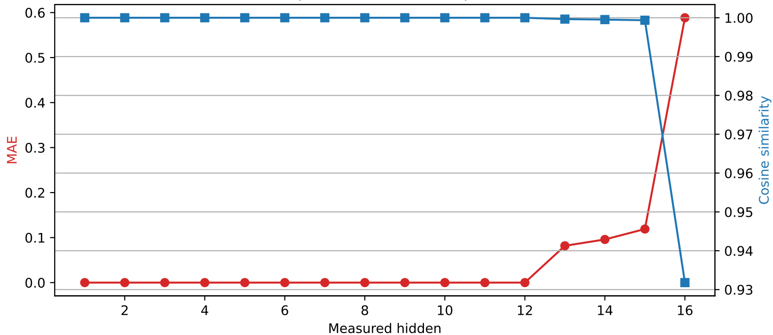
Llama-3.2-1B | Quantized layer 12 | float16 \rightarrow int4
