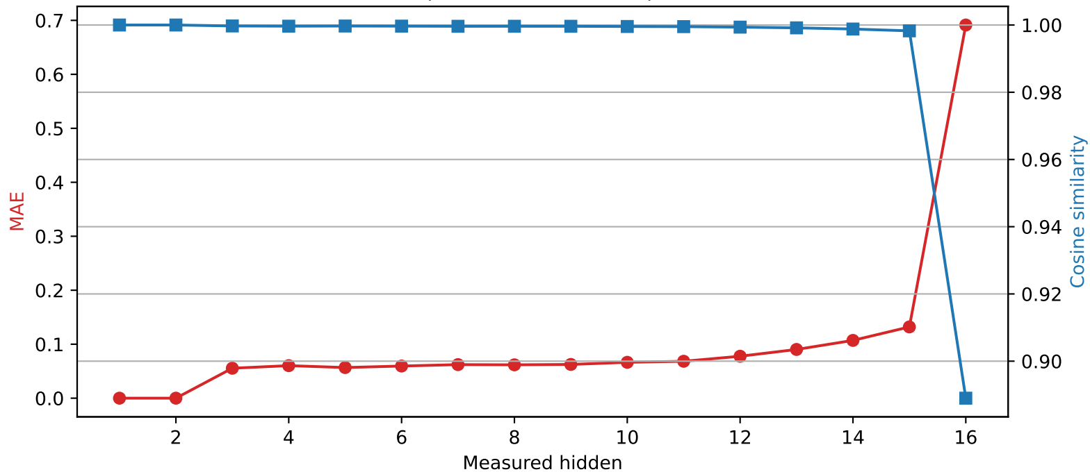
Llama-3.2-1B | Quantized layer 2 | float16 \rightarrow int4
