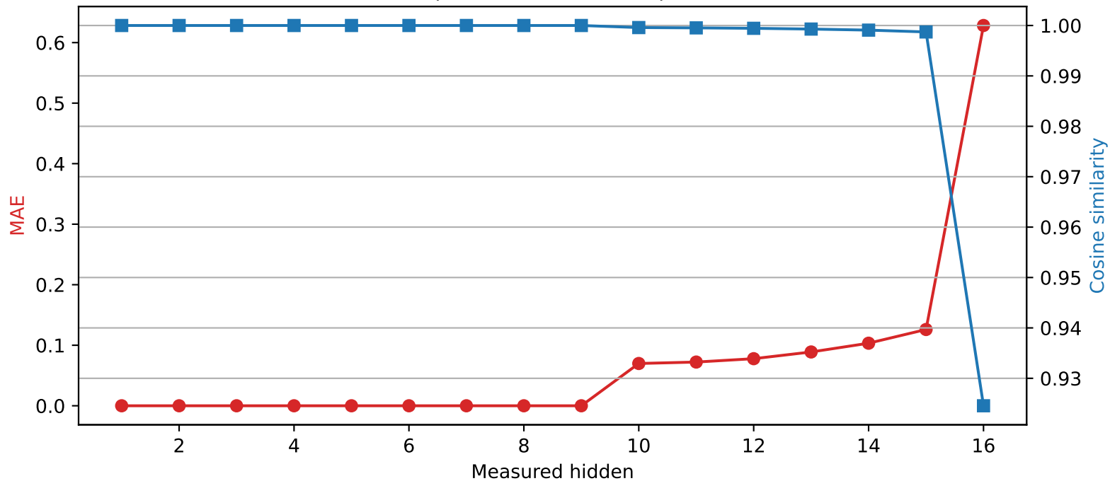
Llama-3.2-1B | Quantized layer 9 | float16 \rightarrow int4
