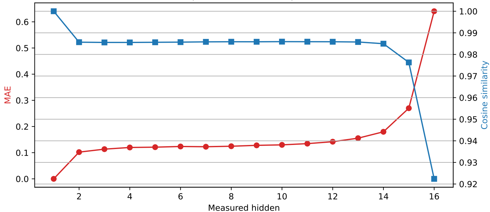
Llama-3.2-1B | Quantized layer 1 | float16 \rightarrow int4
