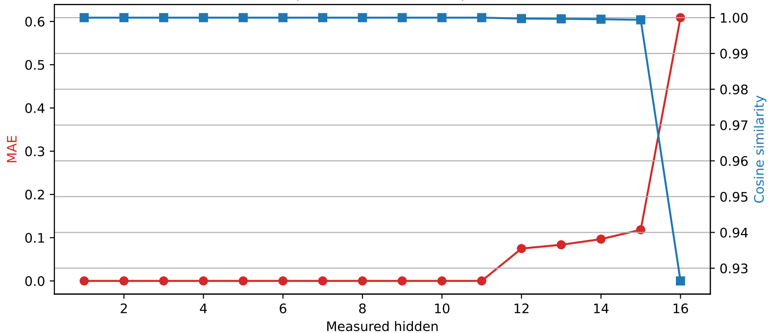
Llama-3.2-1B | Quantized layer 11 | float32 \rightarrow int4
