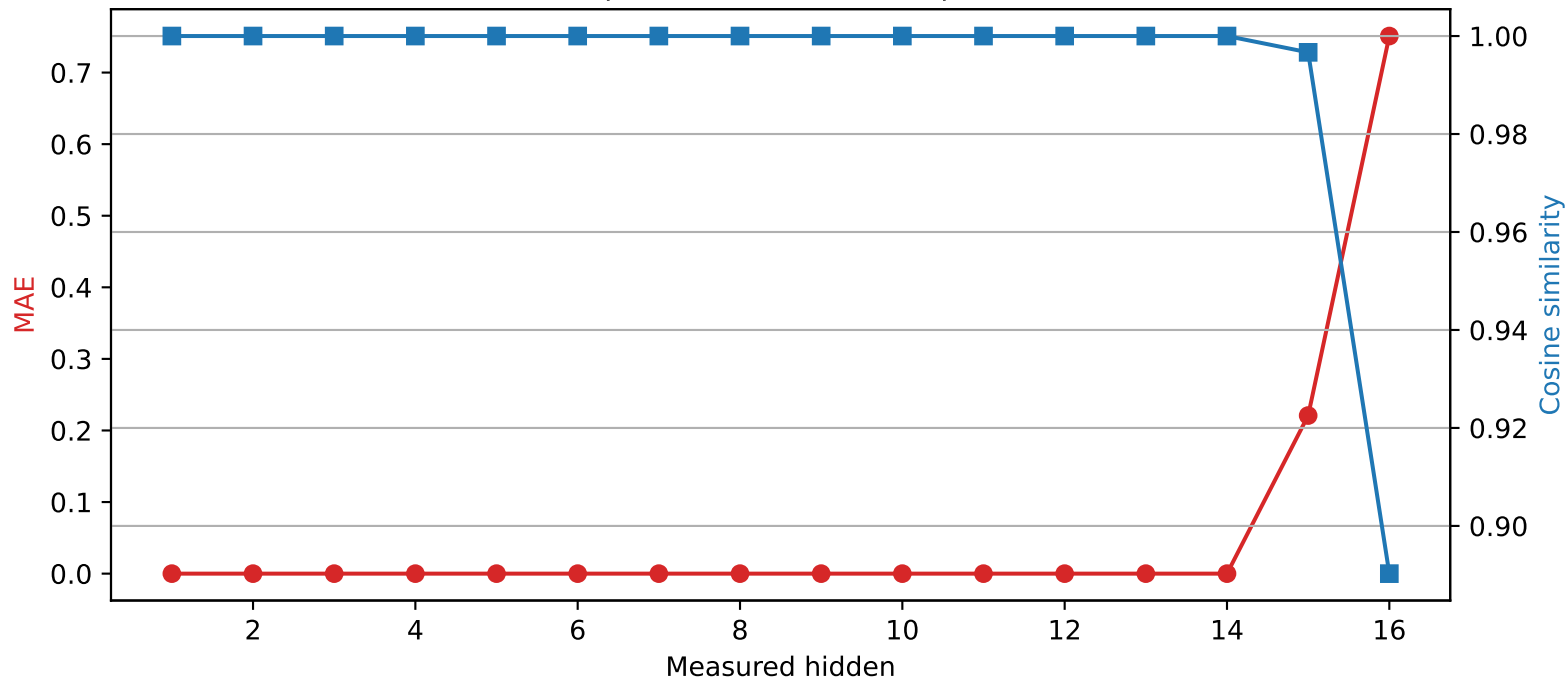
Llama-3.2-1B | Quantized layer 14 | float32 \rightarrow int4
