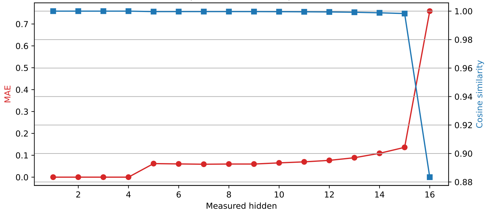
Llama-3.2-1B | Quantized layer 4 | float32 \rightarrow int4
