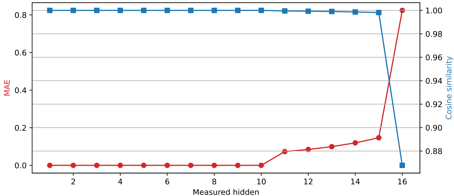
Llama-3.2-1B | Quantized layer 10 | float32 \rightarrow int4
