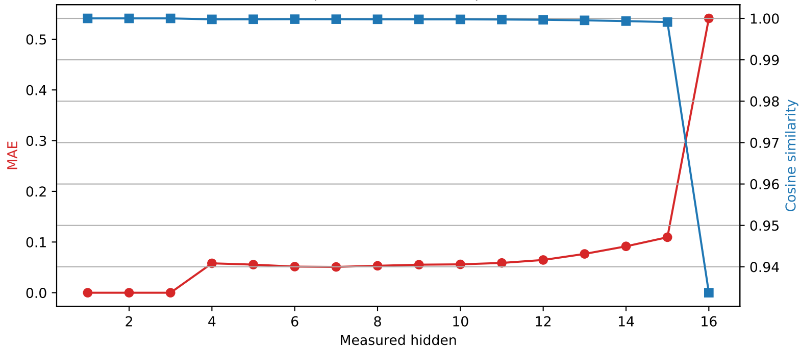
Llama-3.2-1B | Quantized layer 3 | float32 \rightarrow int4
