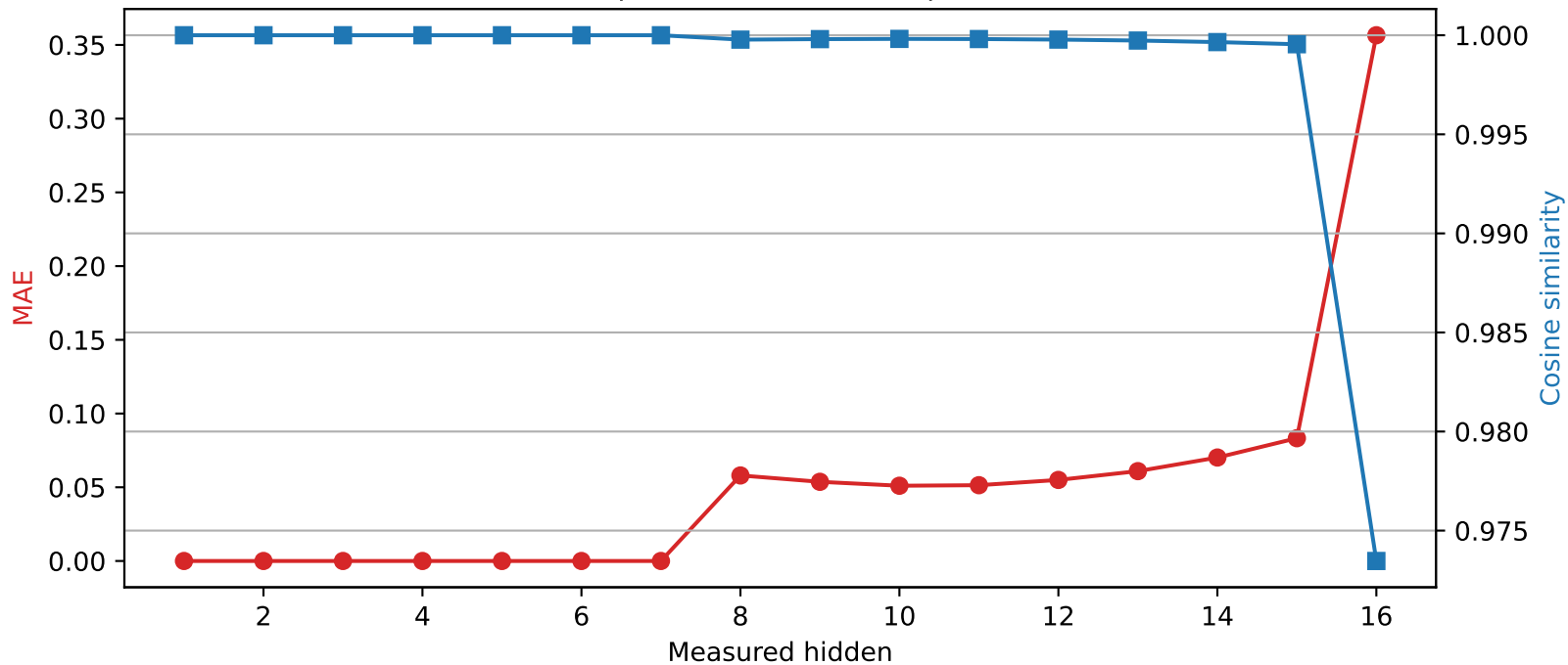
Llama-3.2-1B | Quantized layer 7 | float32 \rightarrow int4
