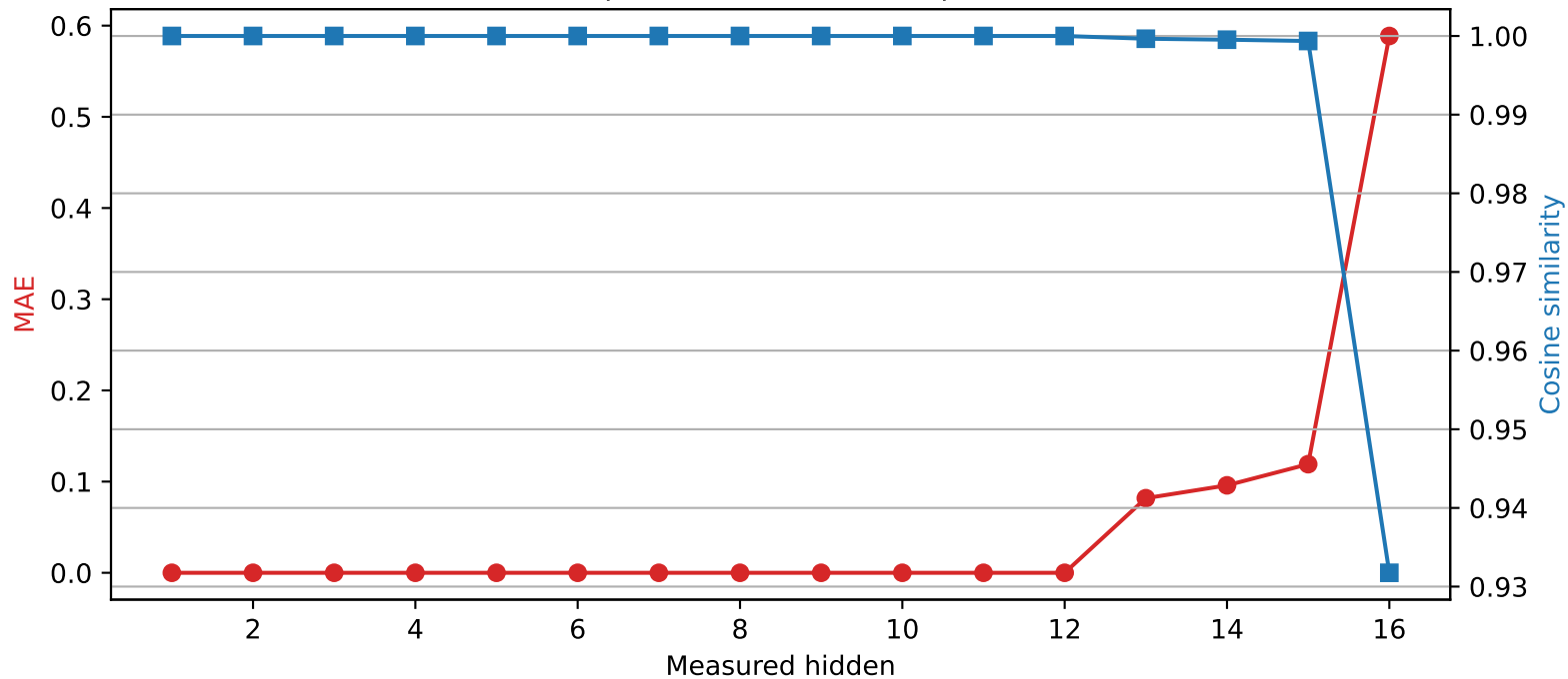
Llama-3.2-1B | Quantized layer 12 | float64 \rightarrow int4
