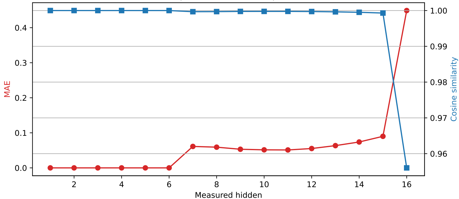
Llama-3.2-1B | Quantized layer 6 | float64 \rightarrow int4
