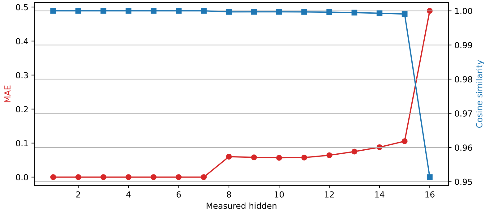
Llama-3.2-1B | Quantized layer 7 | float64 \rightarrow int4
