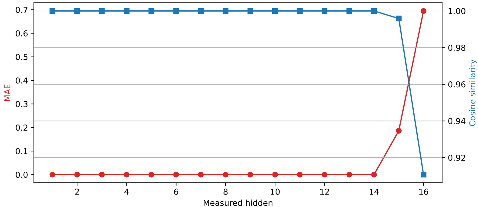
Llama-3.2-1B | Quantized layer 14 | float64 \rightarrow int4
