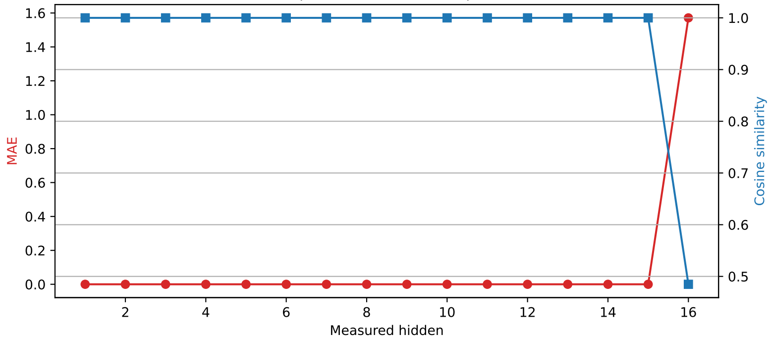
Llama-3.2-1B | Quantized layer 15 | float64 \rightarrow int4
