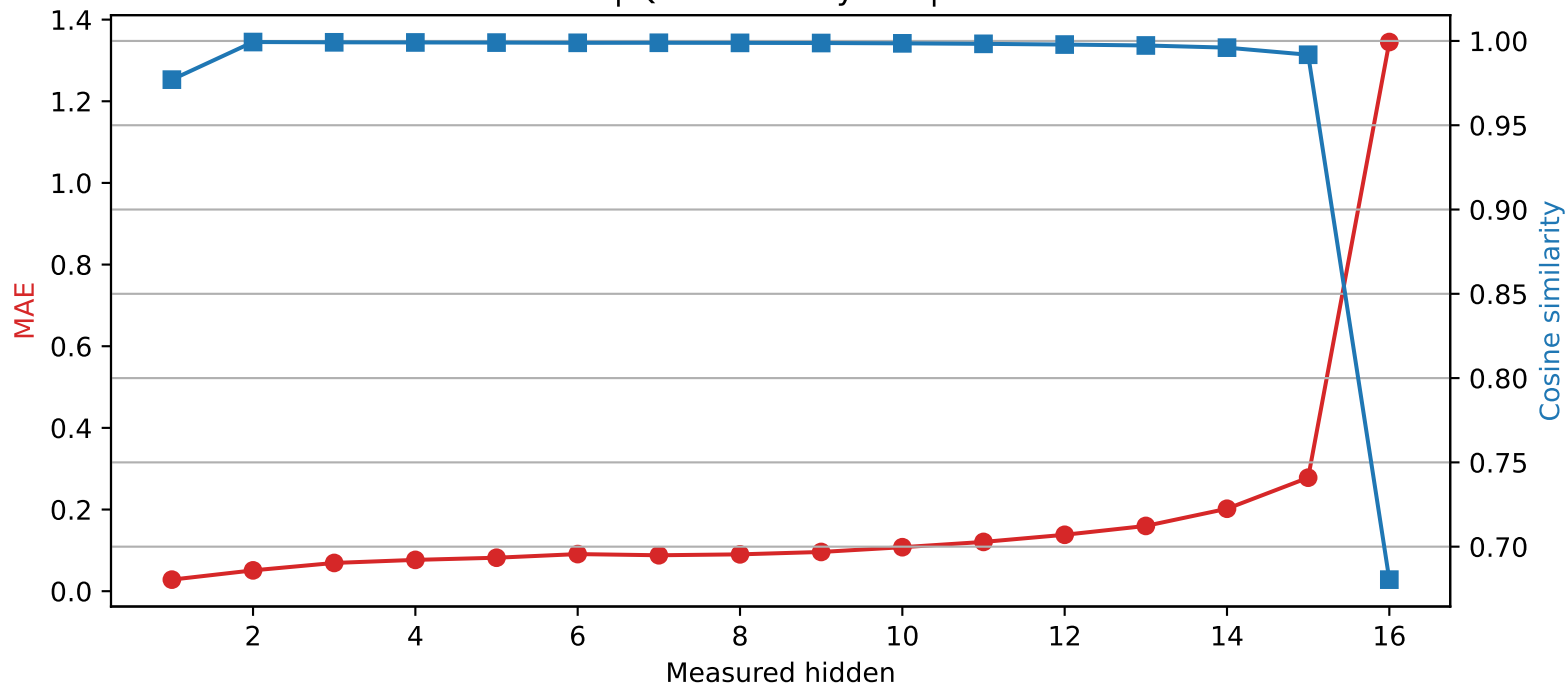
Llama-3.2-1B | Quantized layer 0 | float64 \rightarrow int4
