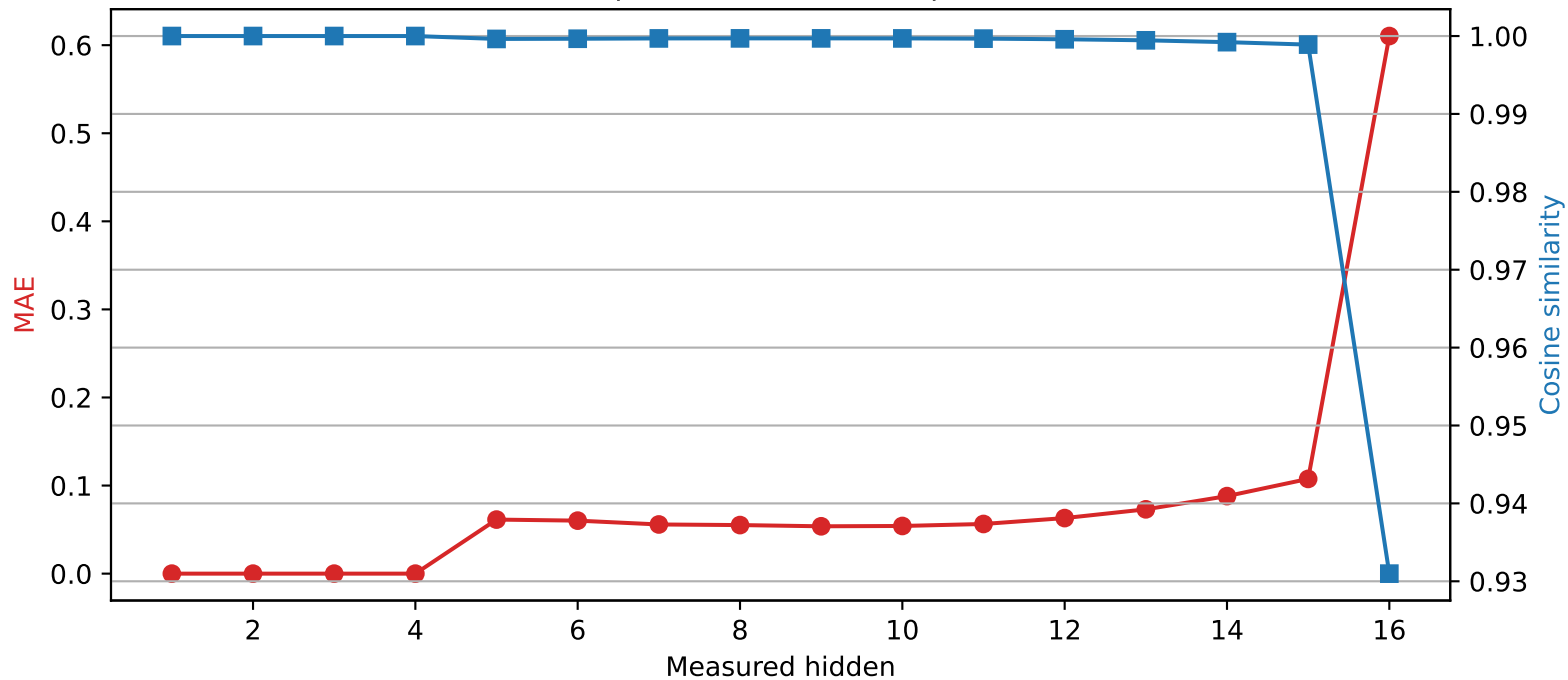
Llama-3.2-1B | Quantized layer 4 | float64 \rightarrow int4
