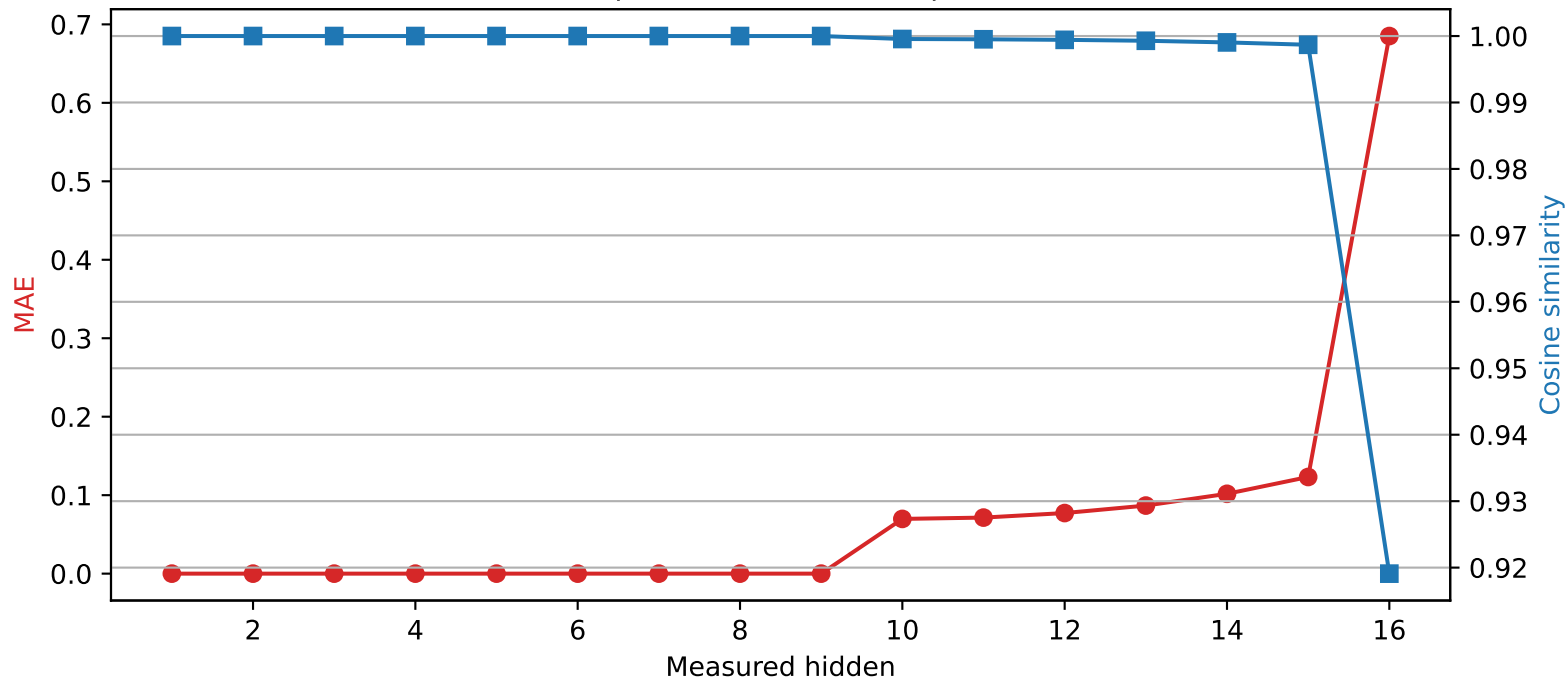
Llama-3.2-1B | Quantized layer 9 | float64 \rightarrow int4
