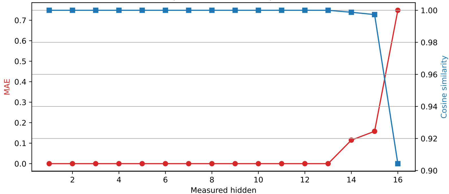
Llama-3.2-1B | Quantized layer 13 | float64 \rightarrow int4
