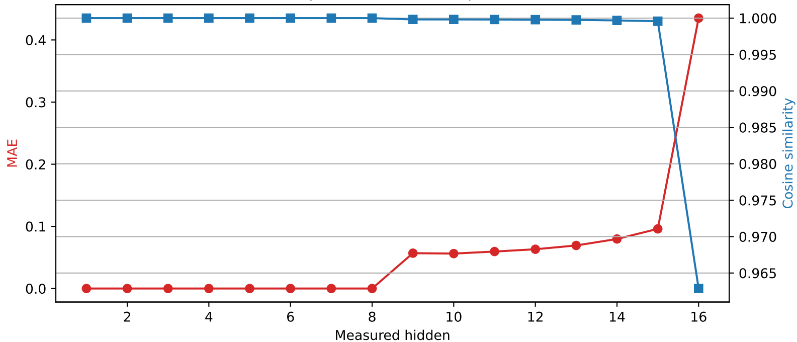
Llama-3.2-1B | Quantized layer 8 | float16 \rightarrow int2
