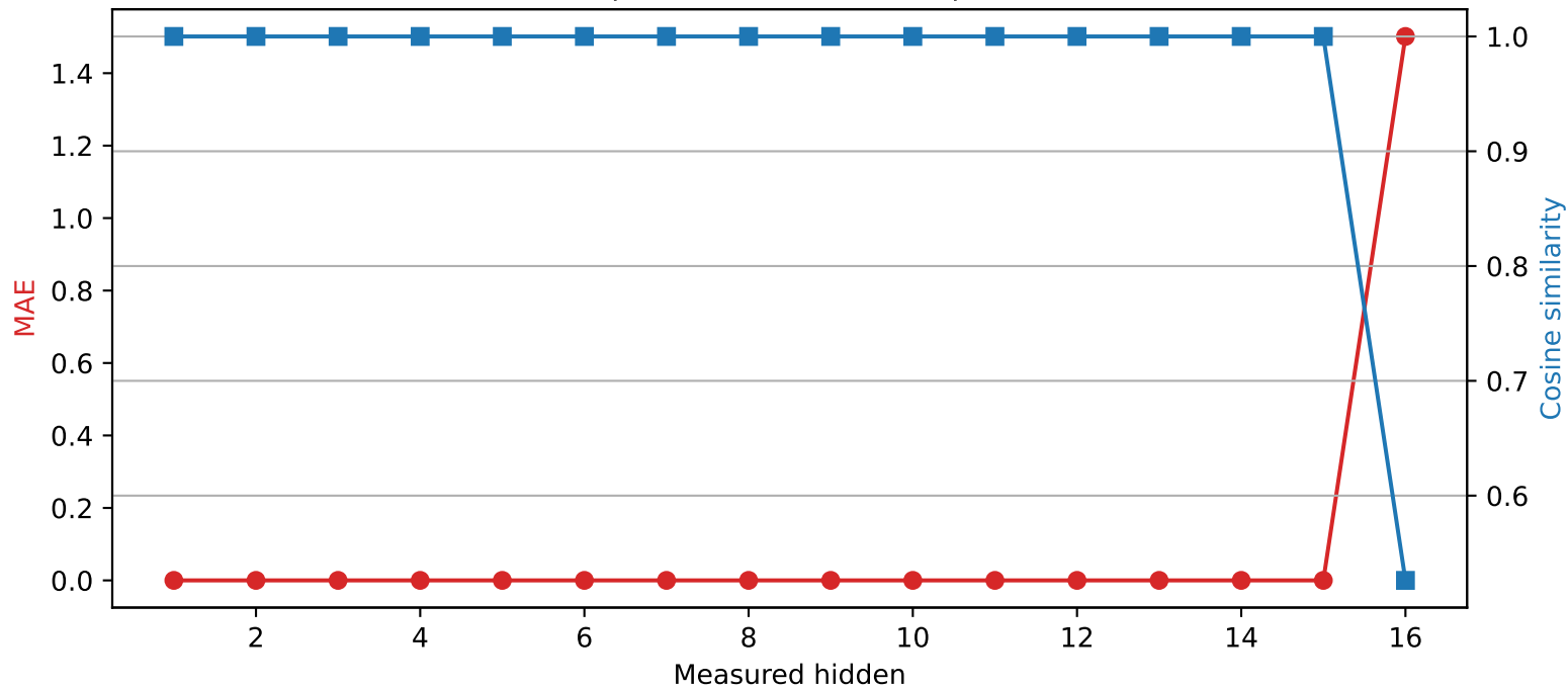
Llama-3.2-1B | Quantized layer 15 | float16 \rightarrow int2
