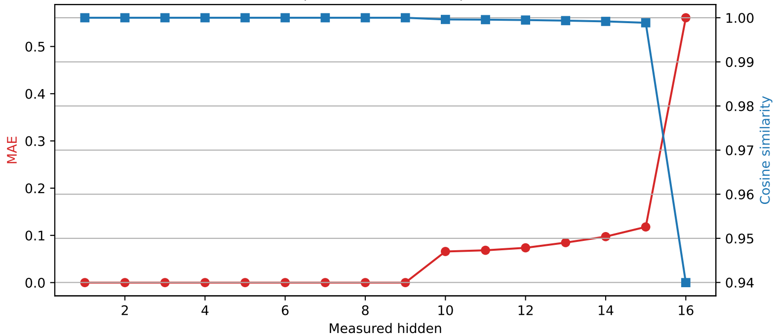
Llama-3.2-1B | Quantized layer 9 | float16 \rightarrow int2
