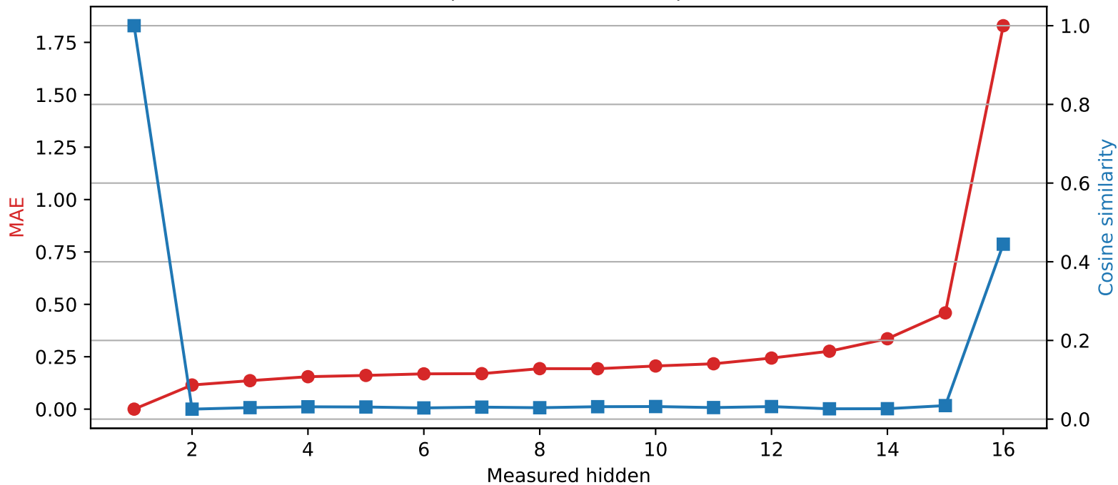
Llama-3.2-1B | Quantized layer 1 | float16 \rightarrow int2
