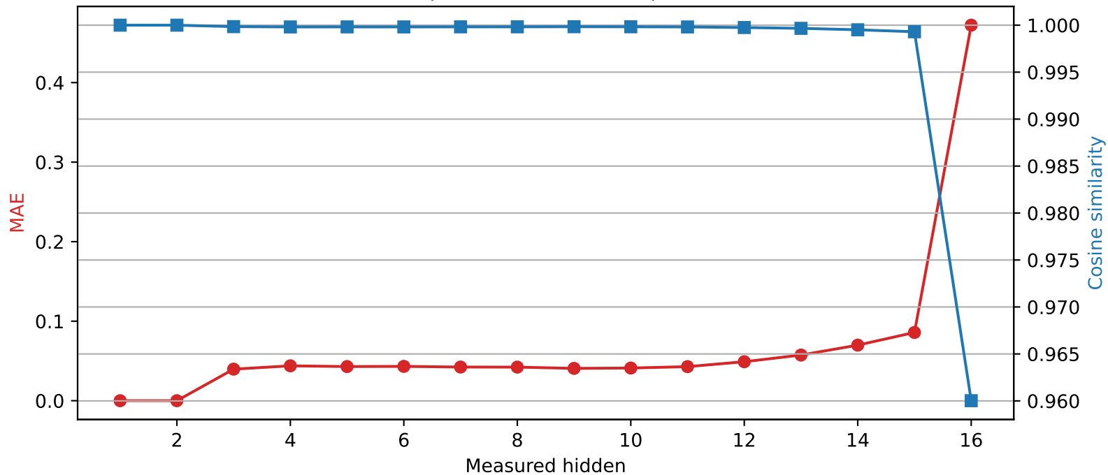
Llama-3.2-1B | Quantized layer 2 | float16 \rightarrow int2
