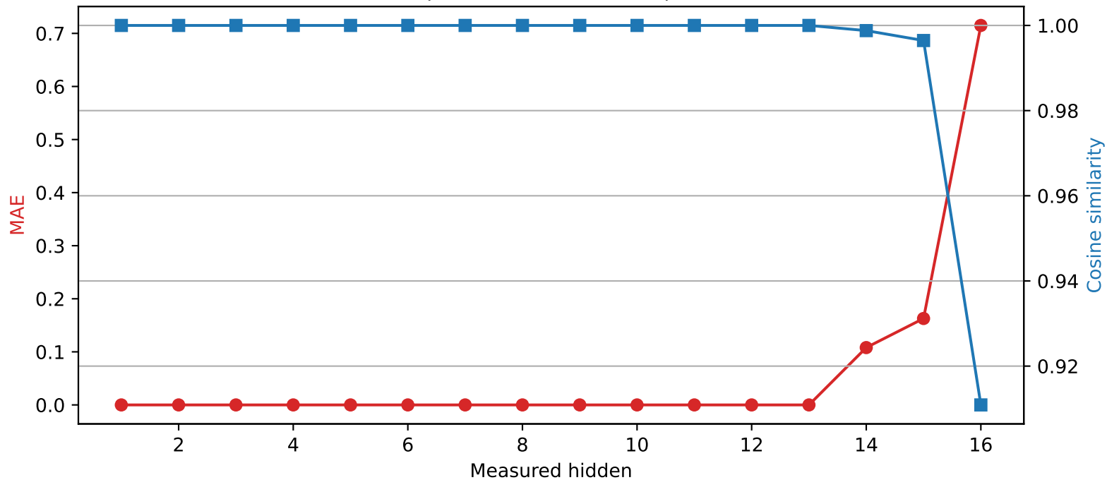
Llama-3.2-1B | Quantized layer 13 | float16 \rightarrow int2
