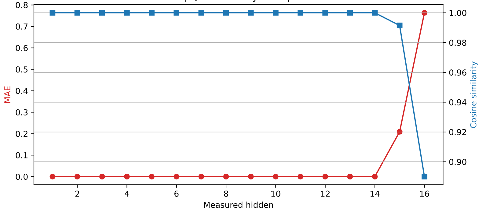
Llama-3.2-1B | Quantized layer 14 | float16 \rightarrow int2
