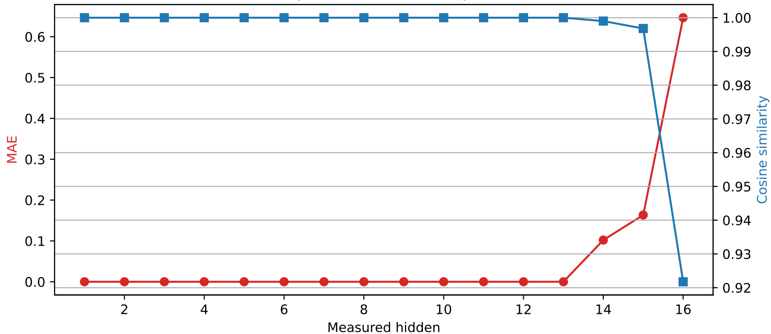
Llama-3.2-1B | Quantized layer 13 | float32 \rightarrow int2
