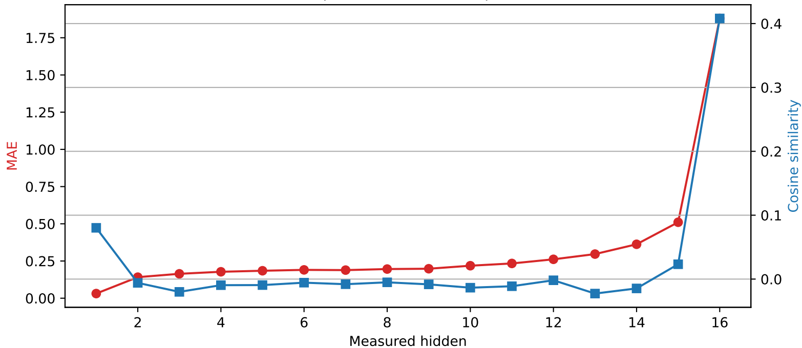
Llama-3.2-1B | Quantized layer 0 | float32 \rightarrow int2
