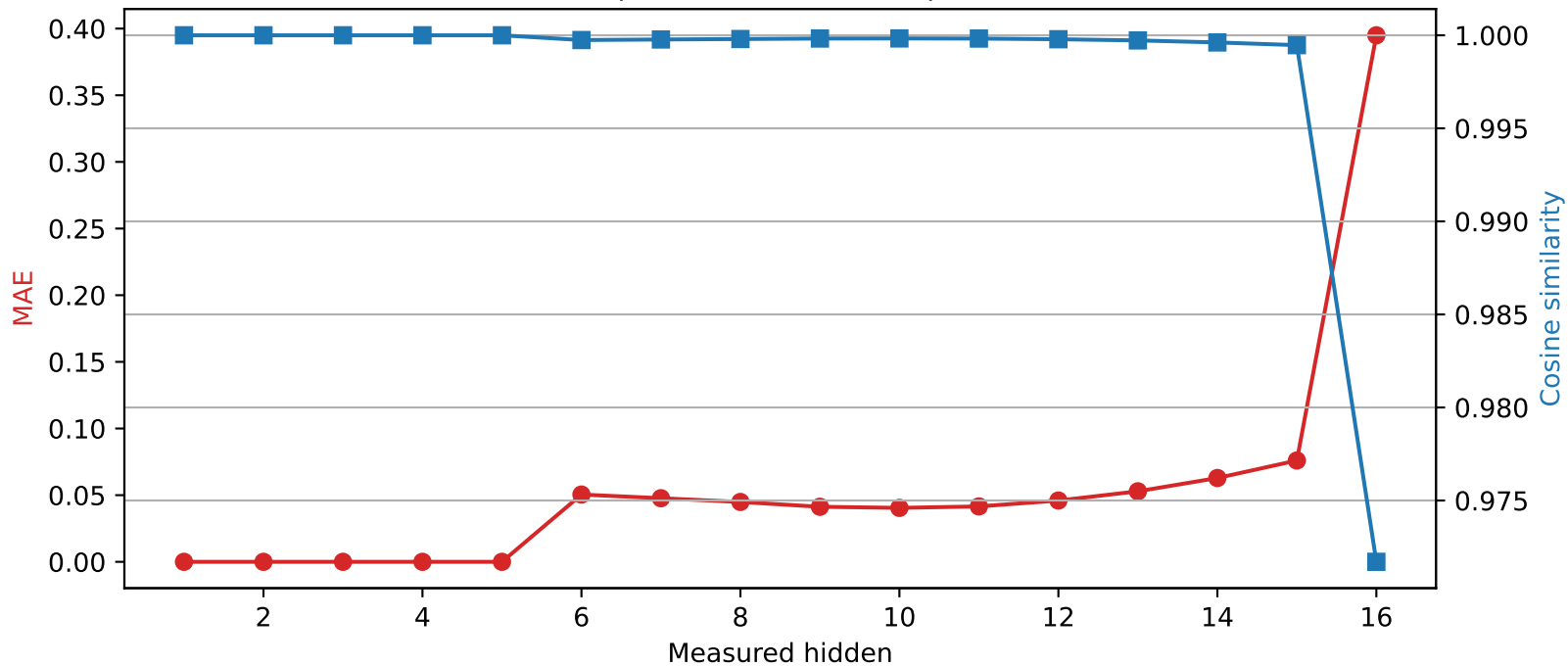
Llama-3.2-1B | Quantized layer 5 | float32 \rightarrow int2
